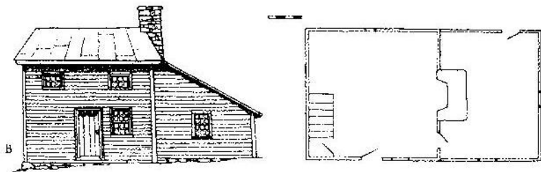
图 A. 位于弗吉尼亚州的格林县靠近胡德市、弗莱彻以南的 V 字形木屋(1963 年 7 月)。至 1966 年 5 月这座木屋已彻底倒塌了。
